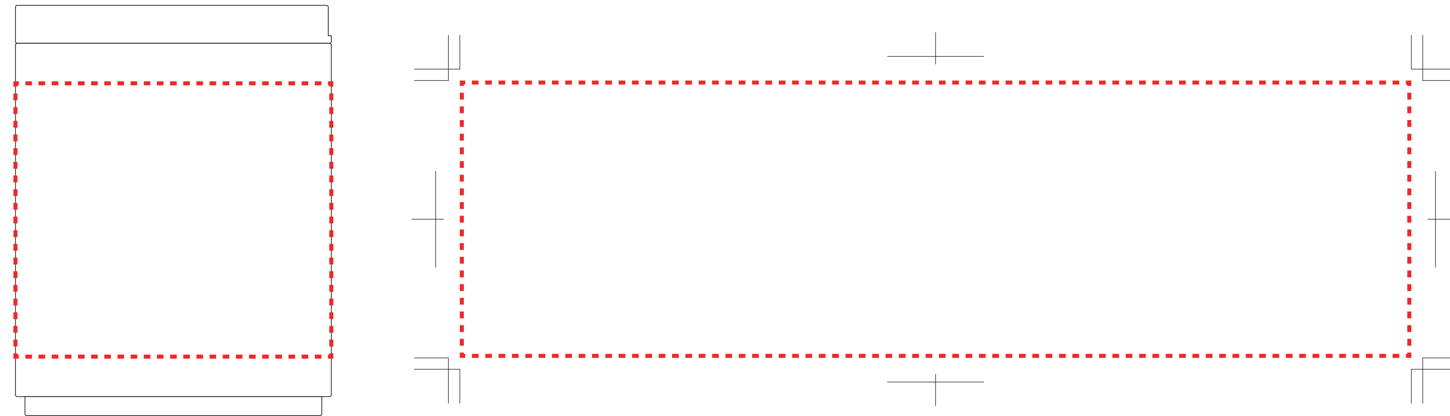
ごはん容器側面（ワイド）：W250×H73mm
