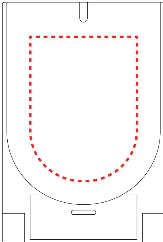
天面(大)：W49×H66mm
