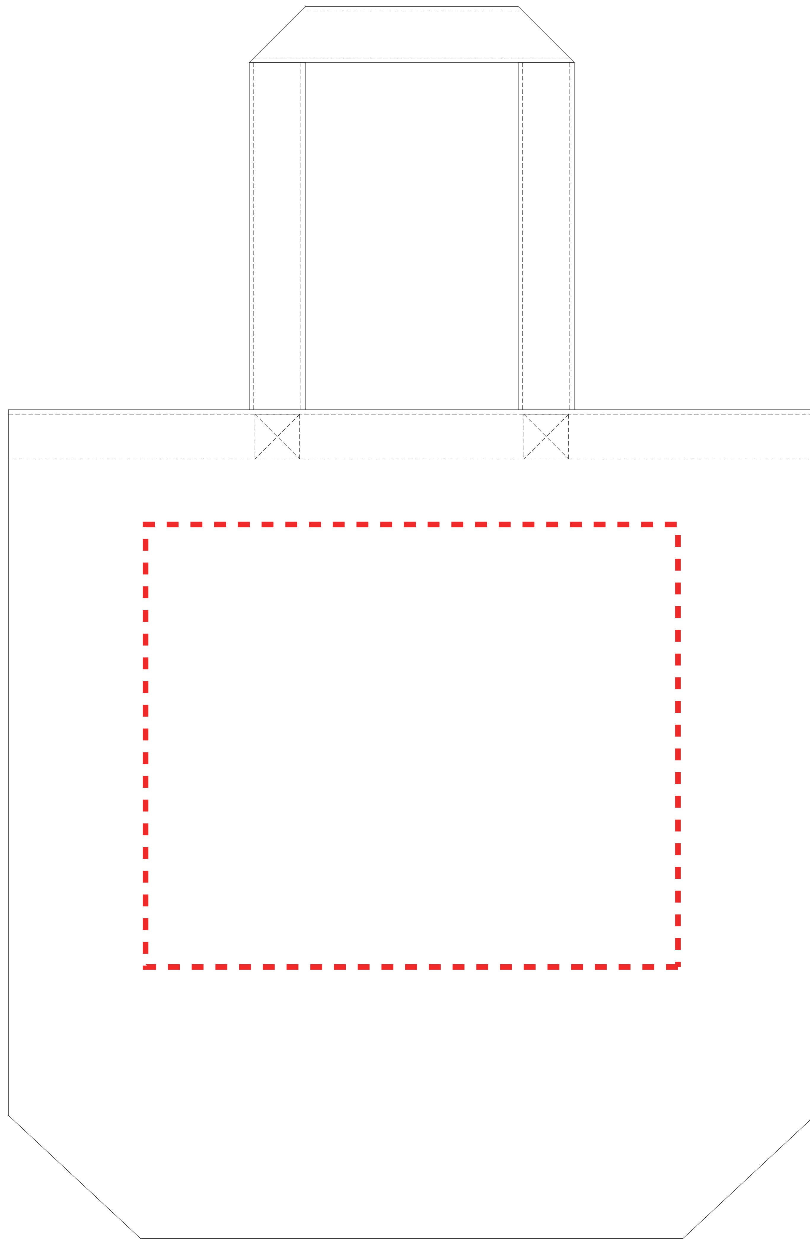
正面：W240×H200mm
